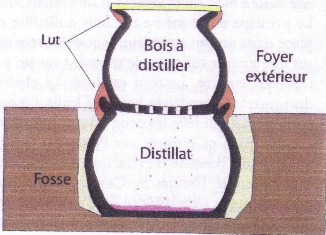
Fig. 7. – Procédé de distillation per descensum selon les traités savants médiévaux (d'après la restitution de N. Thomas).
